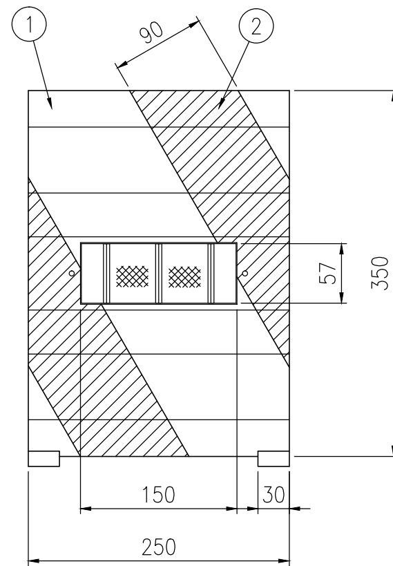
姿図 S=1/5
