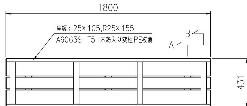
平面図(S=1/20)
