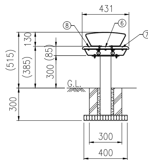
側面図(S=1/20)
