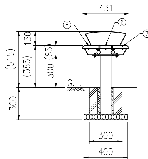
側面図(S=1/20)
