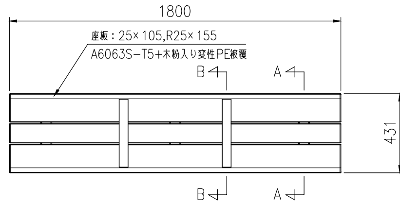
平面図(S=1/20)
