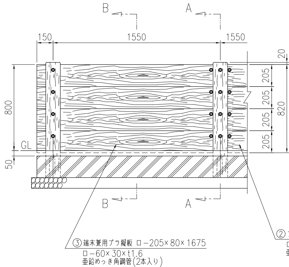
C部詳細図 (1/8)
