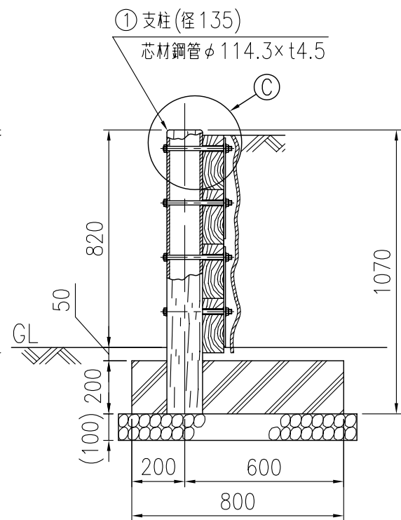
A-A断面図 (1/20)
