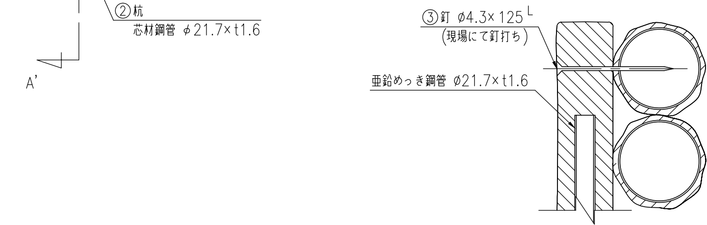
A-A'断面図 (1/4)
