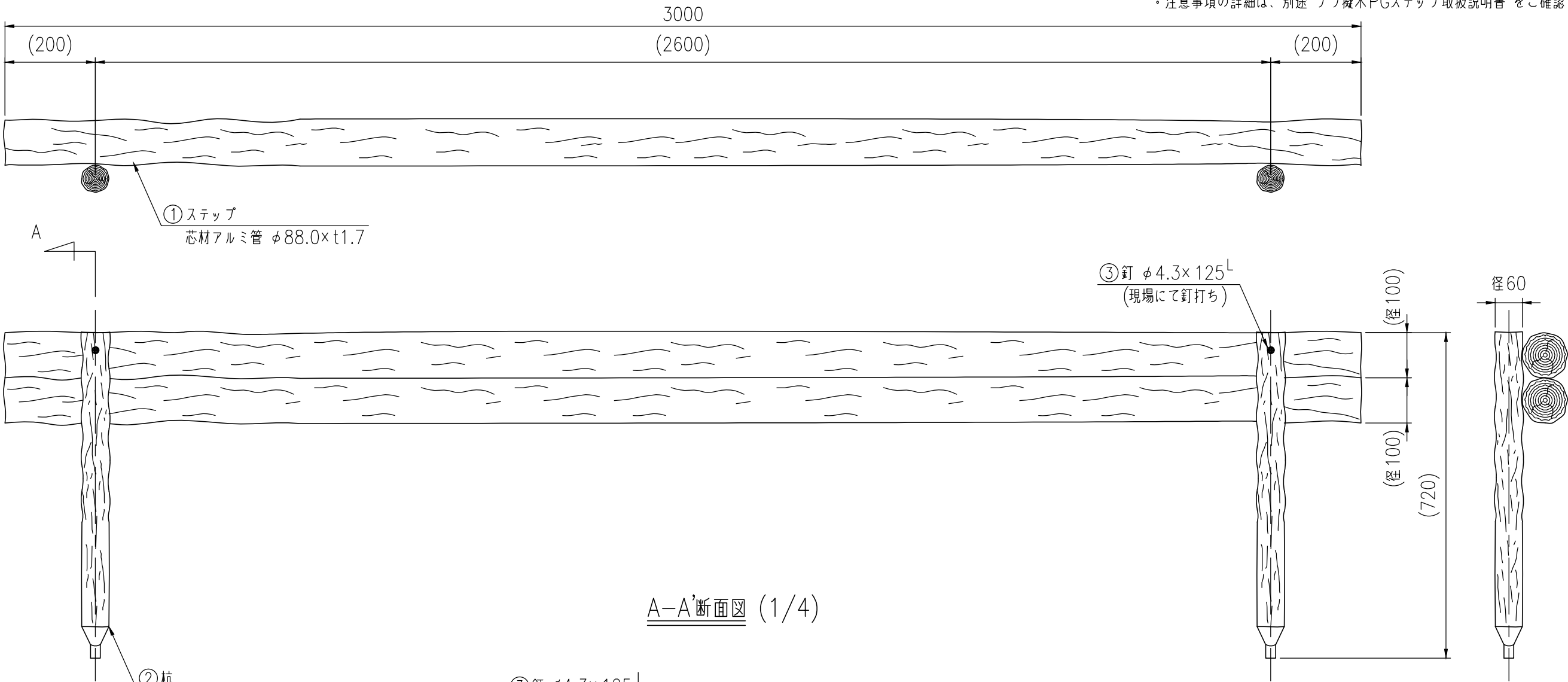
設置図 (1/10)
