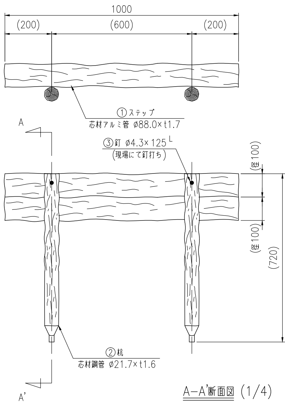
設置図 (1/10)
