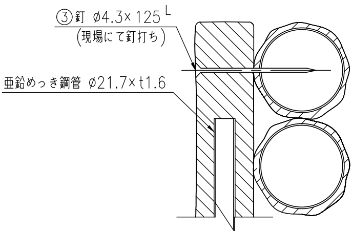
A-A'断面図 (1/4)
