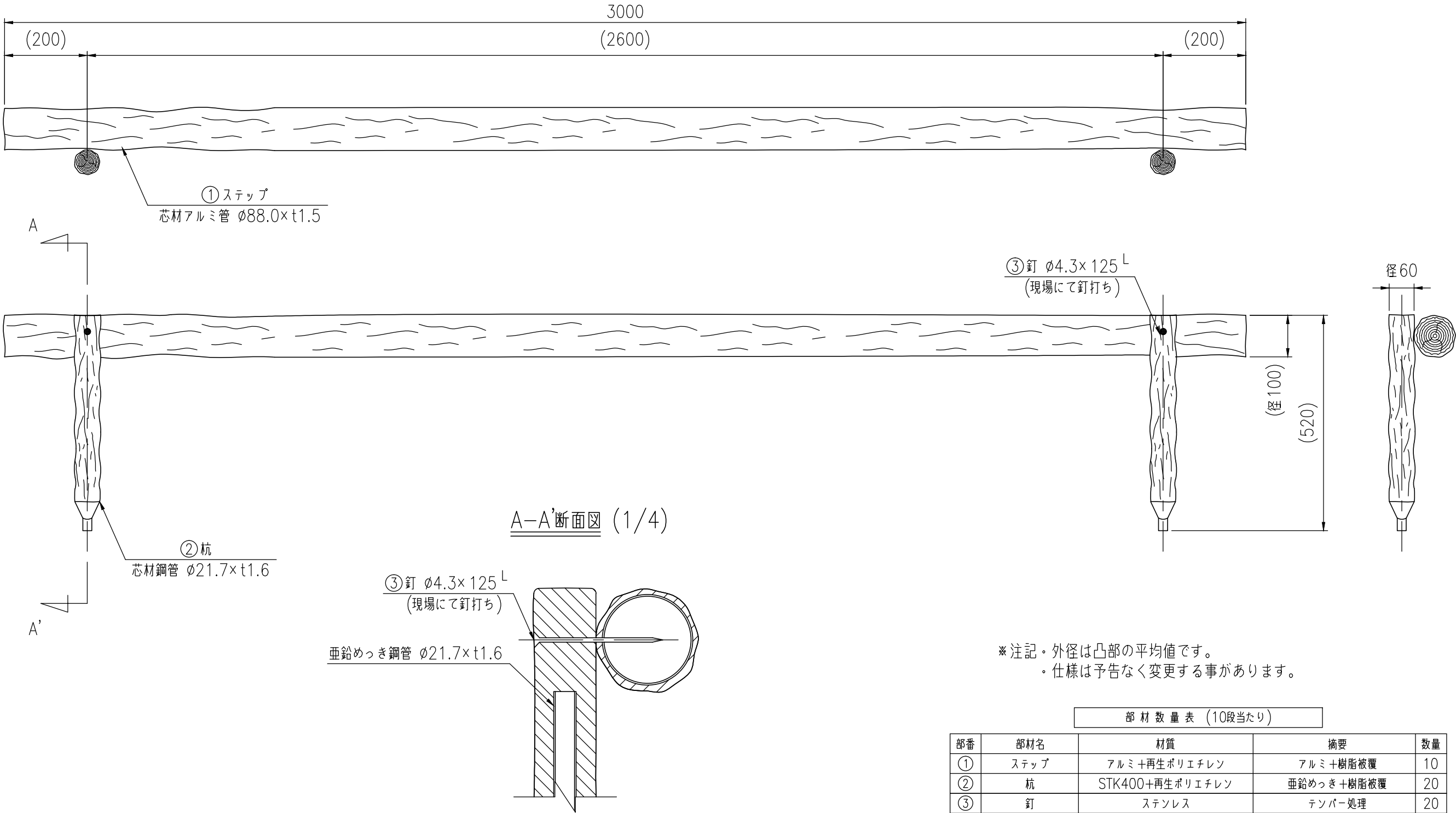
設置図 (1/10)
