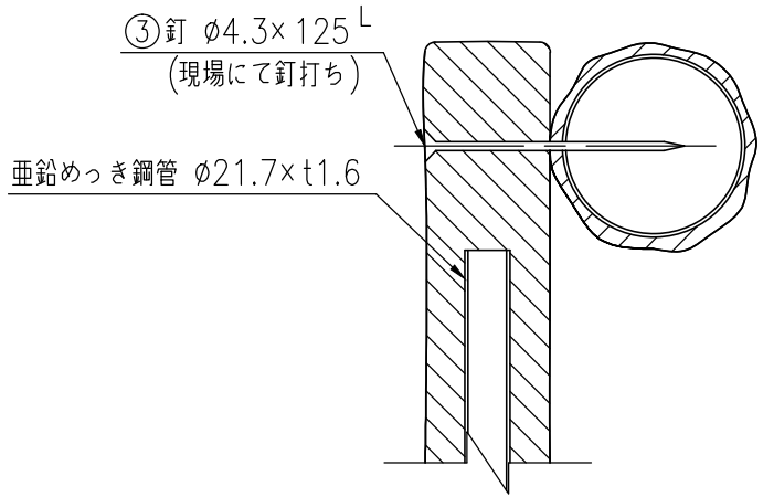
A-A'断面図 (1/4)
