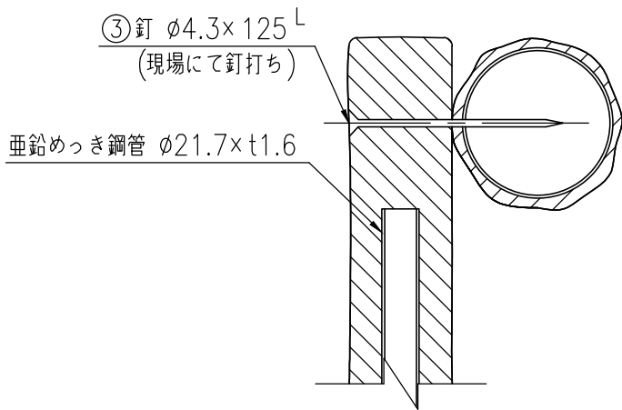
A-A'断面図 (1/4)
