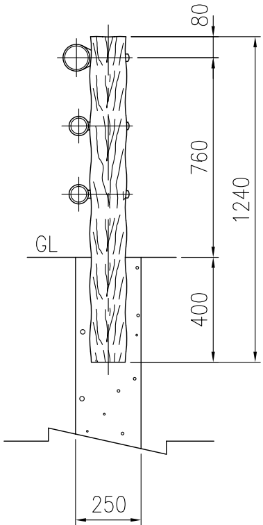
＜連続基礎式＞ P5-PG-308B
