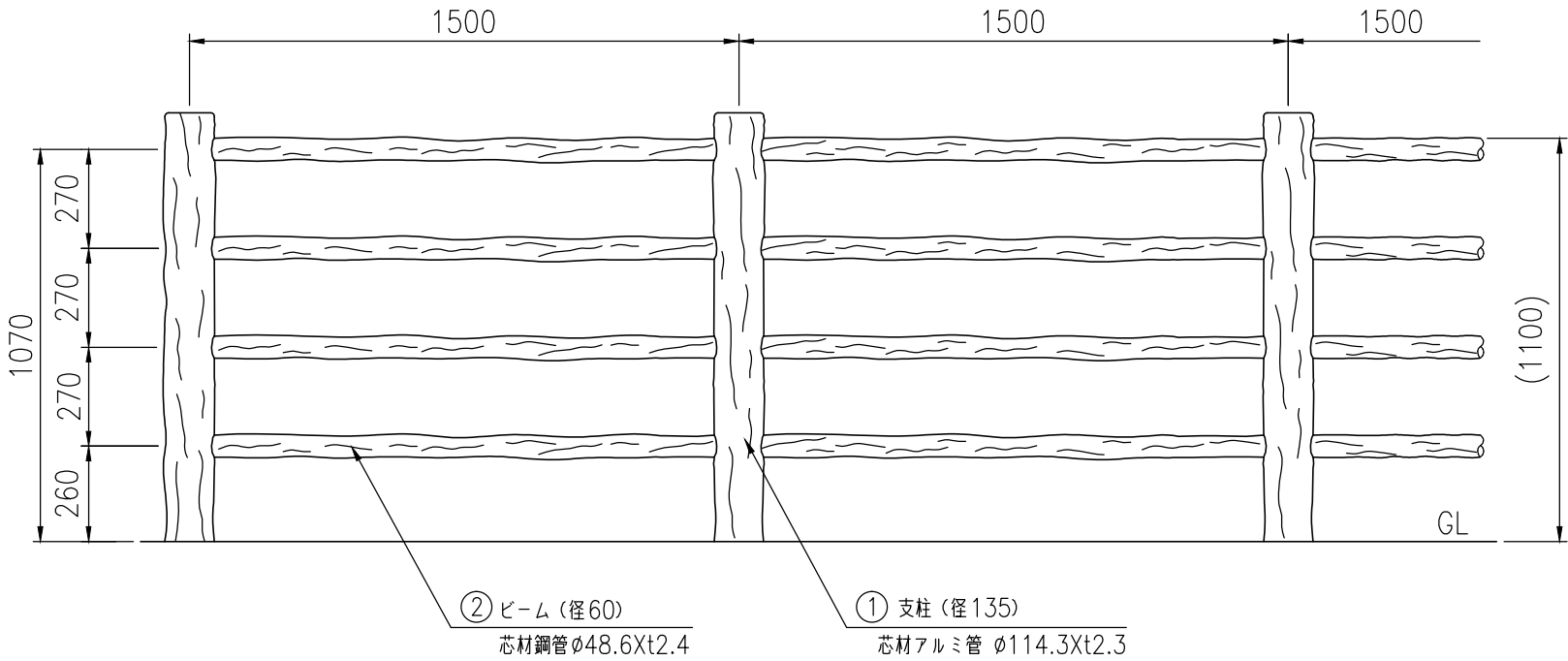
設置図 (1/20)
