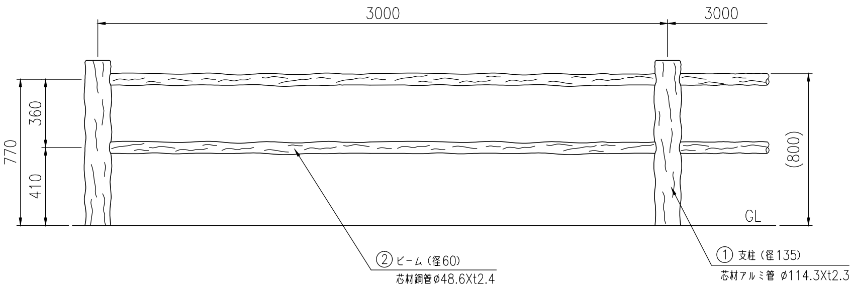
設置図 (1 / 20)
