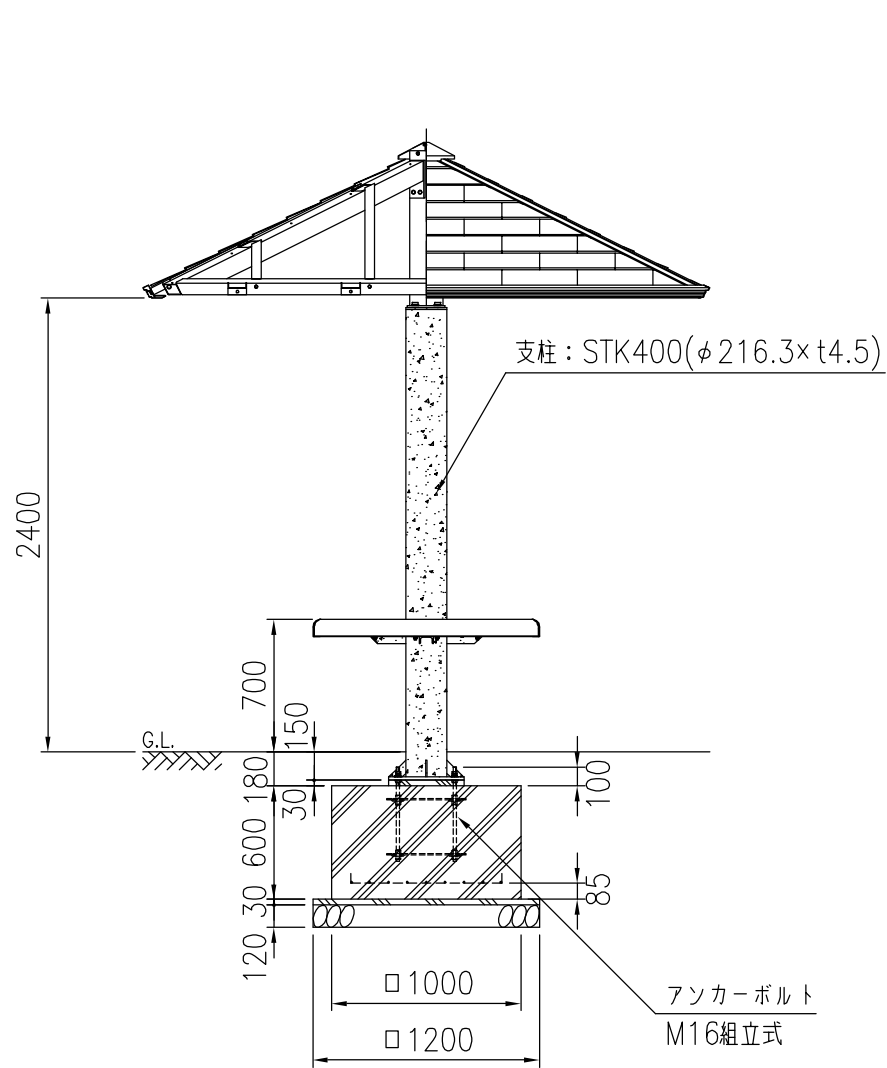
立面・断面図
