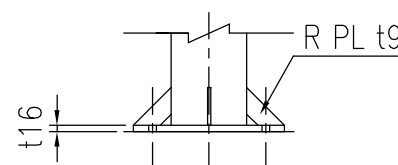
ベースプレート詳細図
