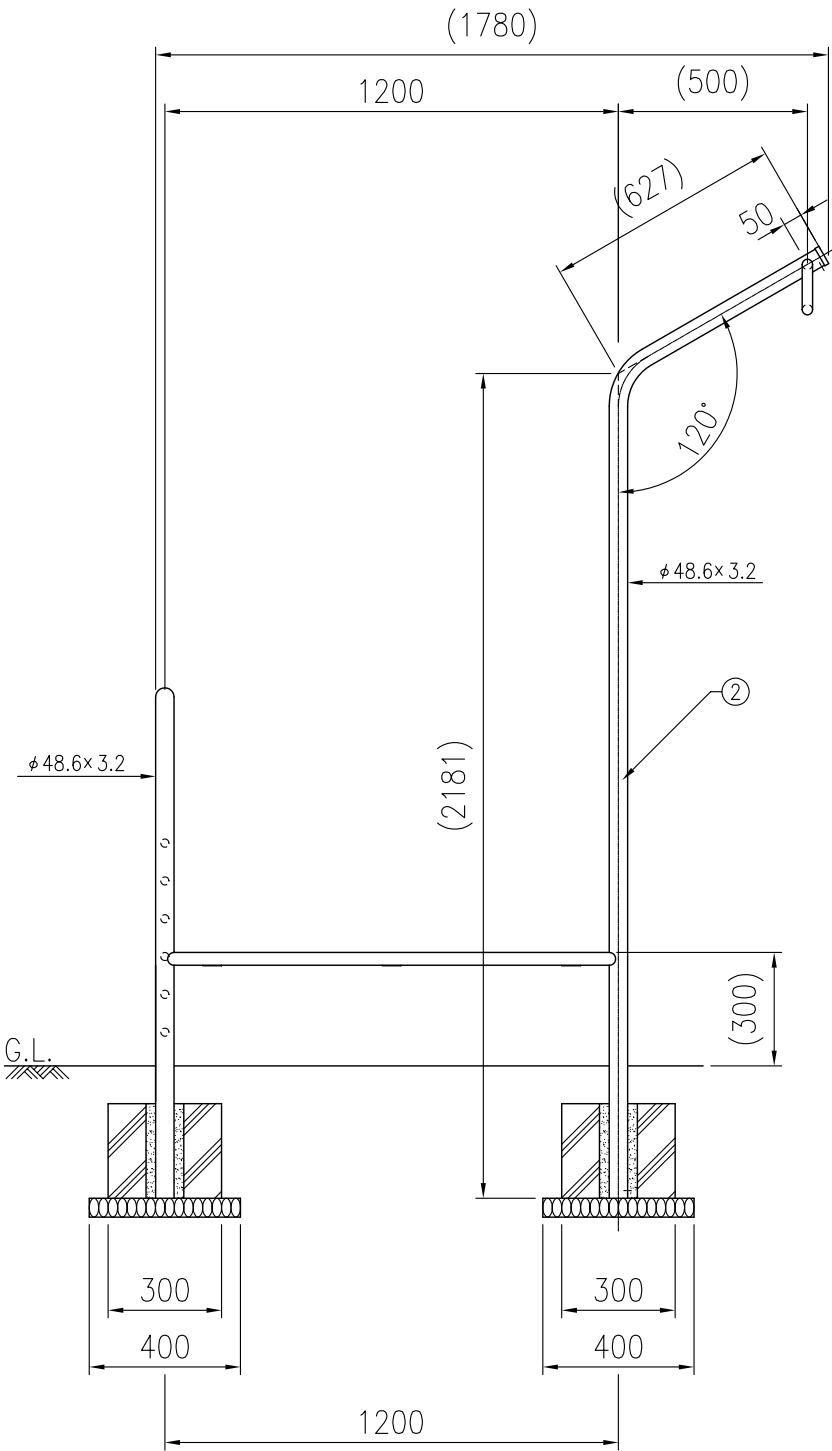
正面図(S=1/20)
