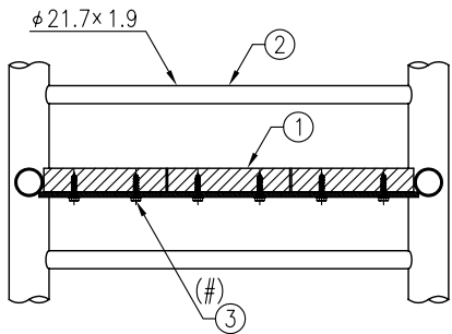
A-A 取付詳細図(S=1/10)
