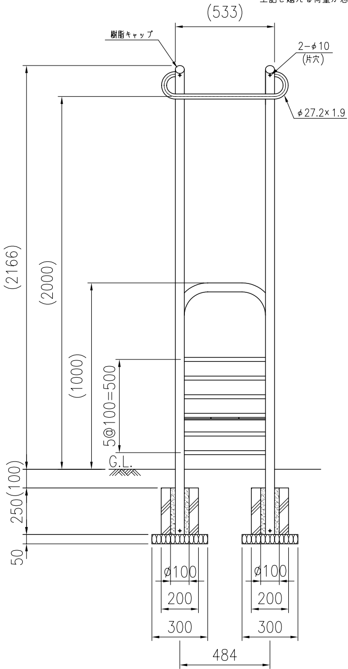
側面図(S=1/20)
