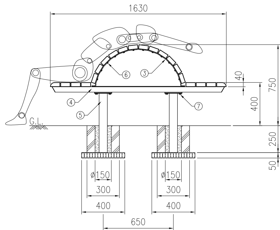
正面図 (S=1/20)
