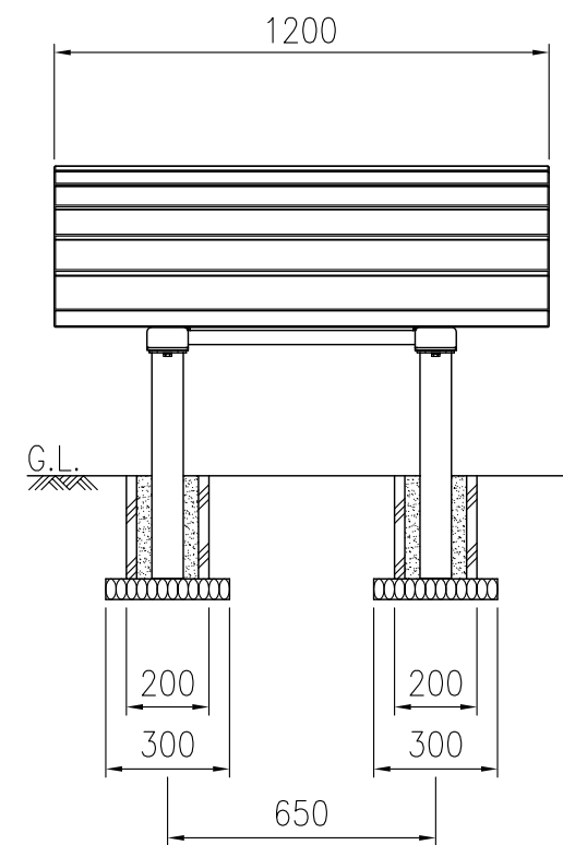
側面図 (S=1/20)
