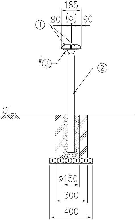
側面図(S=1/20)
