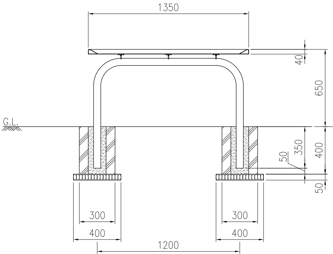
正面図(S=1/20)
