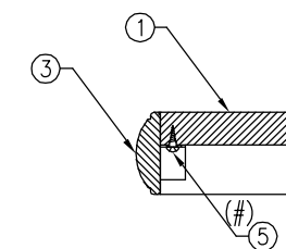
端末キャップ取付詳細図
