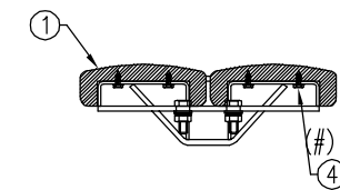
座部取付詳細図(A-A矢視図)(S=1/10)
