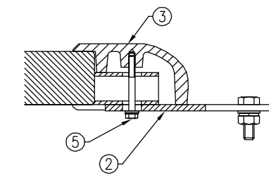
脚部カバー取付詳細図(S=1/5)
