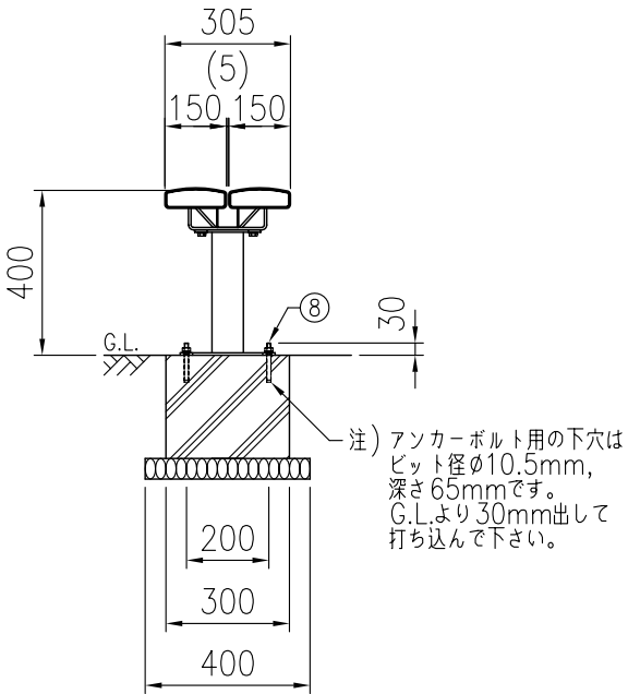
側面図(S=1/20)
