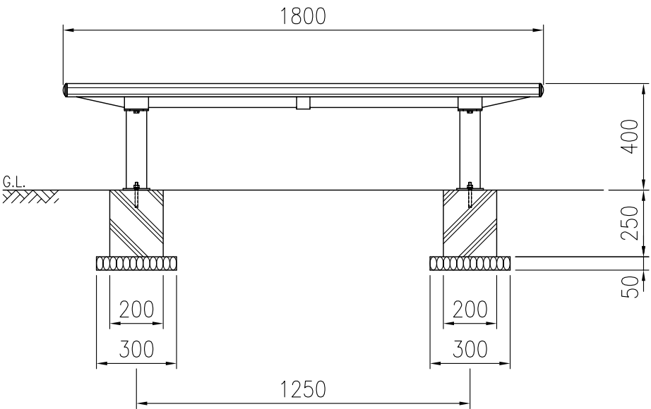
正面図(S=1/20)
