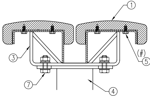
座部取付詳細図 (A-A矢視図)(S=1/5)
