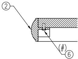
端末キャップ取付詳細図(S=1/5)
