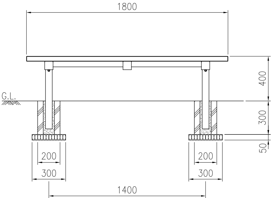
正面図(S=1/20)
