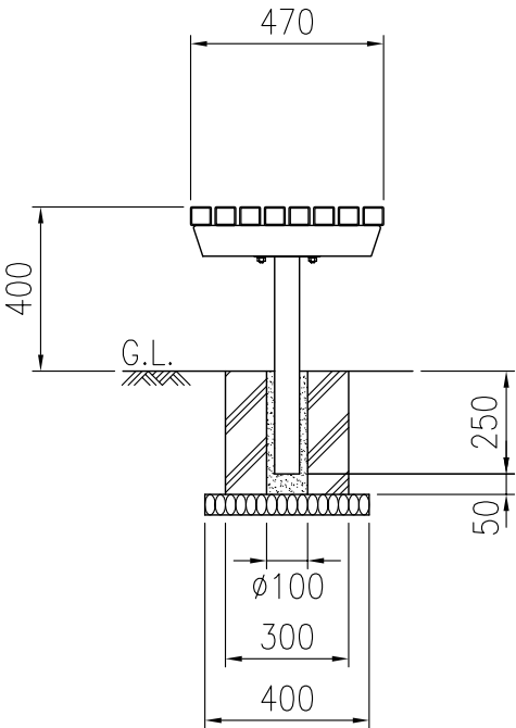
側面図(S=1/20)
