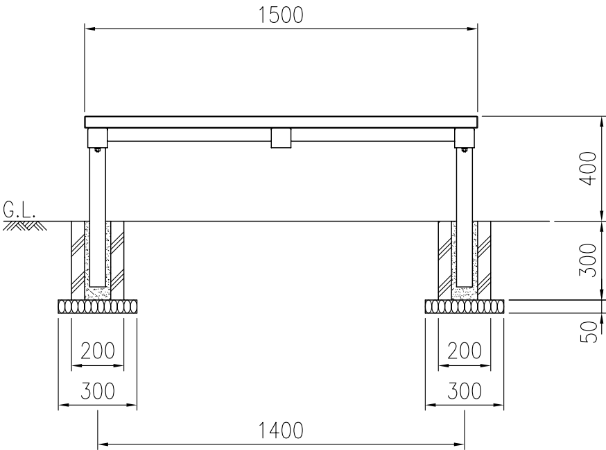
正面図(S=1/20)
