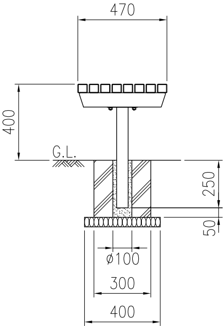
側面図(S=1/20)
