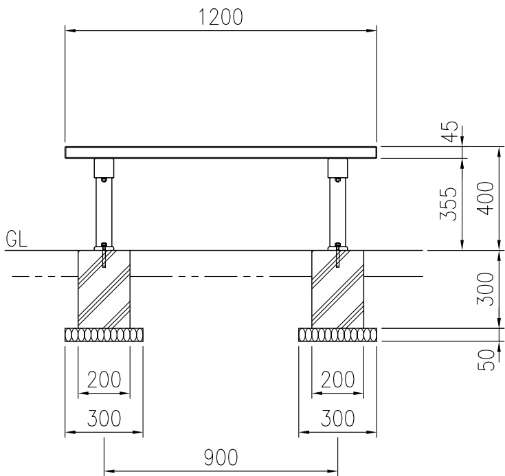
正面図 (S=1/20)
