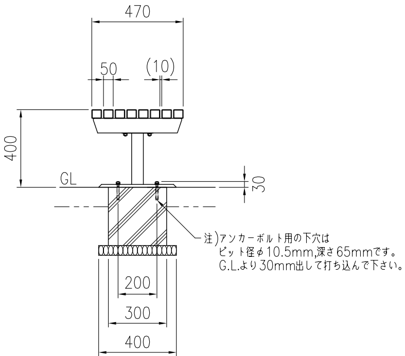
側面図 (S=1/20)
