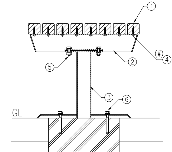
組付断面図 (A-A矢視図) (S=1/10)
