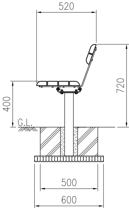
側面図 (S=1/20)
