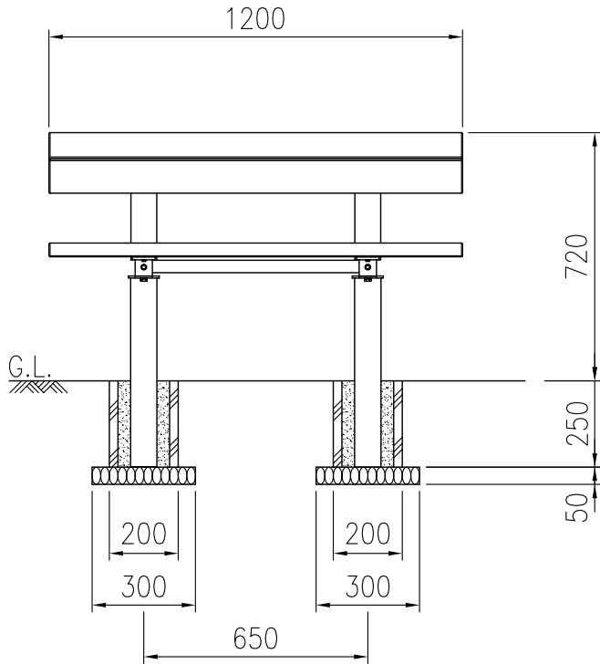
正面図 (S=1/20)
