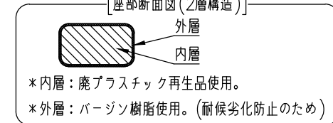
[座部断面図(2層構造)]
