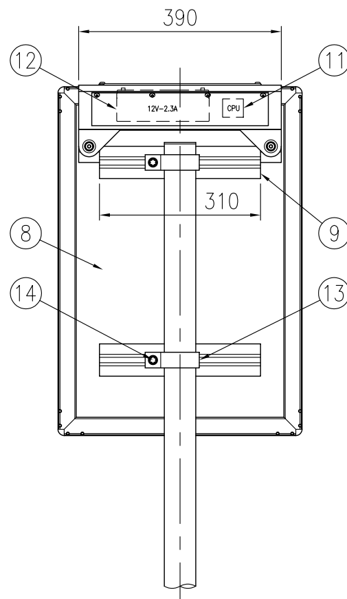
背面図 S=1/10
