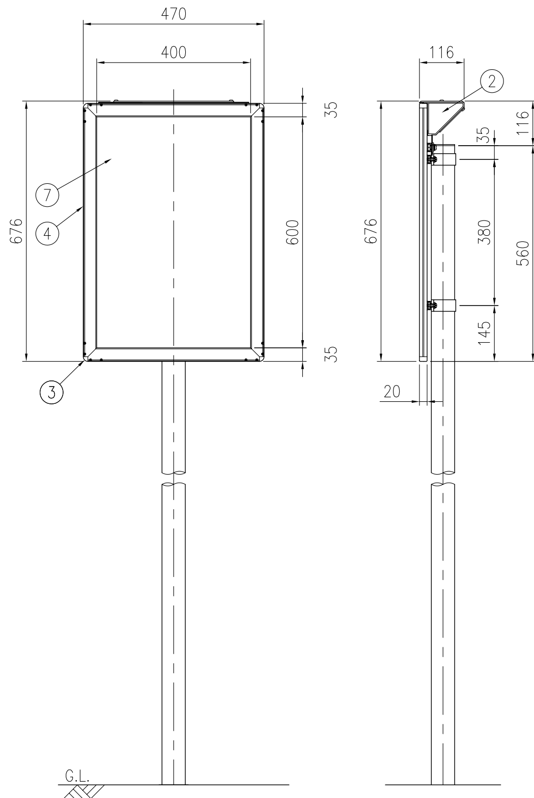
正面図 S=1/10
