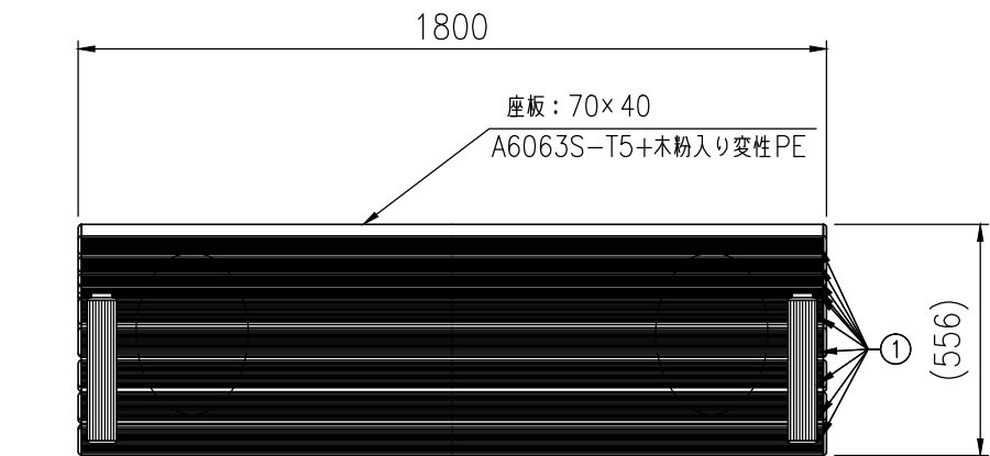
平面図 (S=1/20)
