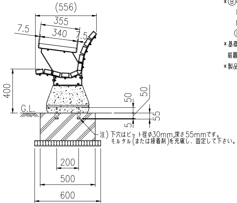
側面図 (S=1/20)
