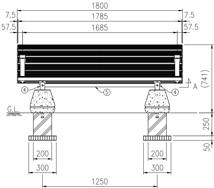
正面図 (S=1/20)
