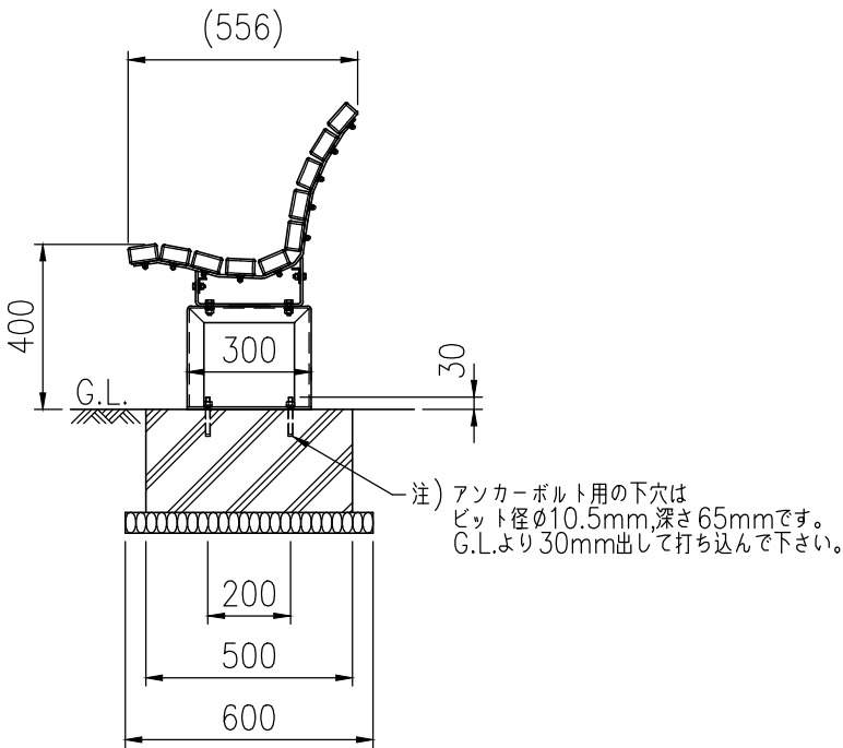
側面図(S=1/20)
