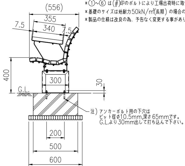
側面図 (S=1/20)
