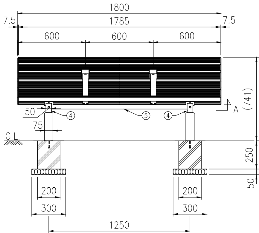
正面図 (S=1/20)
