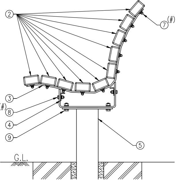
組付詳細図(S=1/10)
