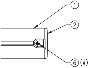
キャップ詳細図(A矢視図)(S=1/5)
