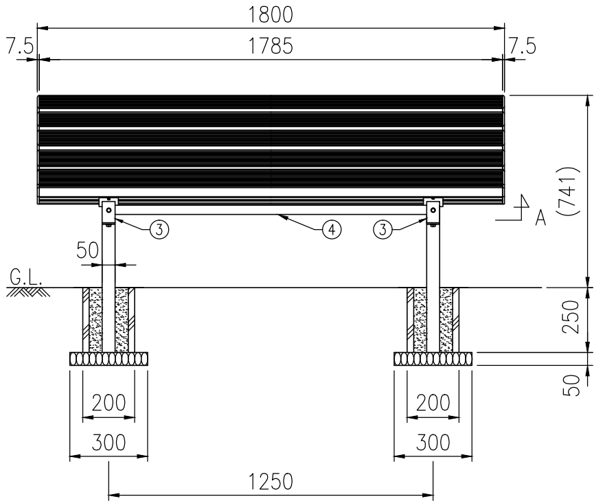
正面図(S=1/20)
