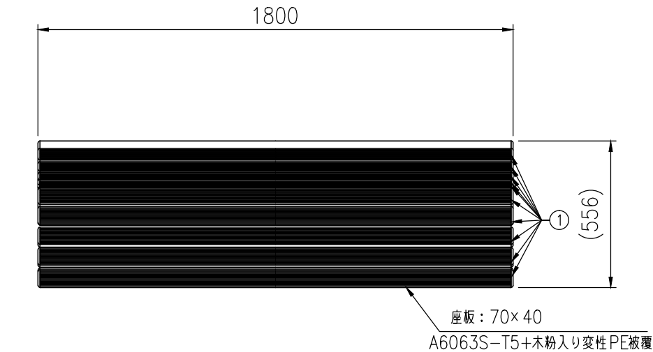
平面図(S=1/20)
