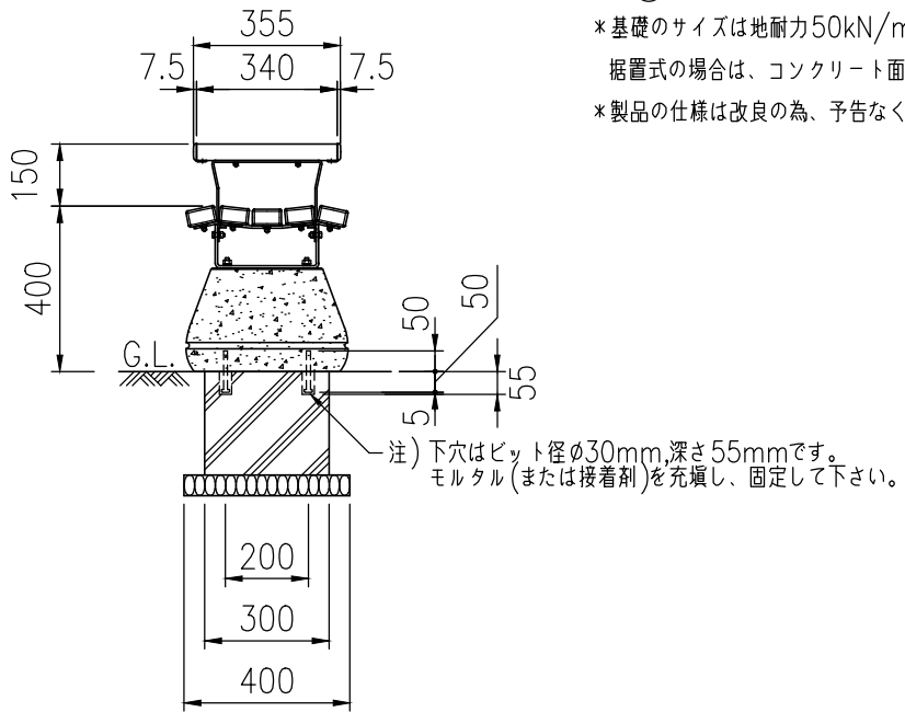
側面図 (S=1/20)
