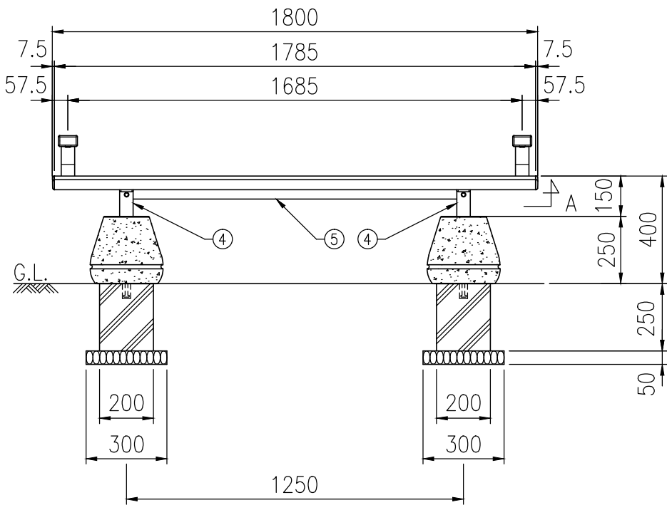
正面図 (S=1/20)
