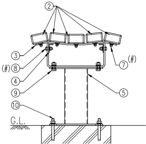
組付詳細図(S=1/10)
