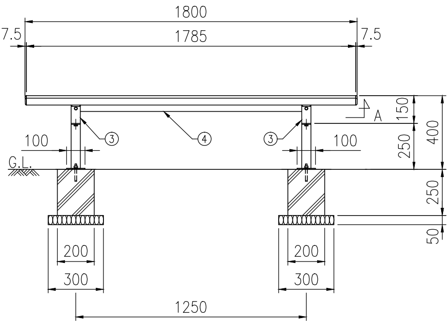
正面図(S=1/20)
