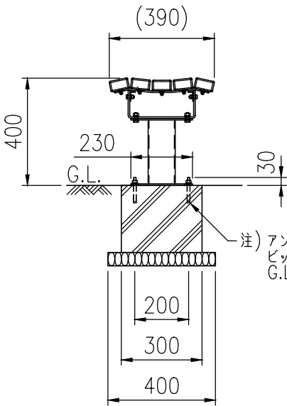
側面図(S=1/20)
