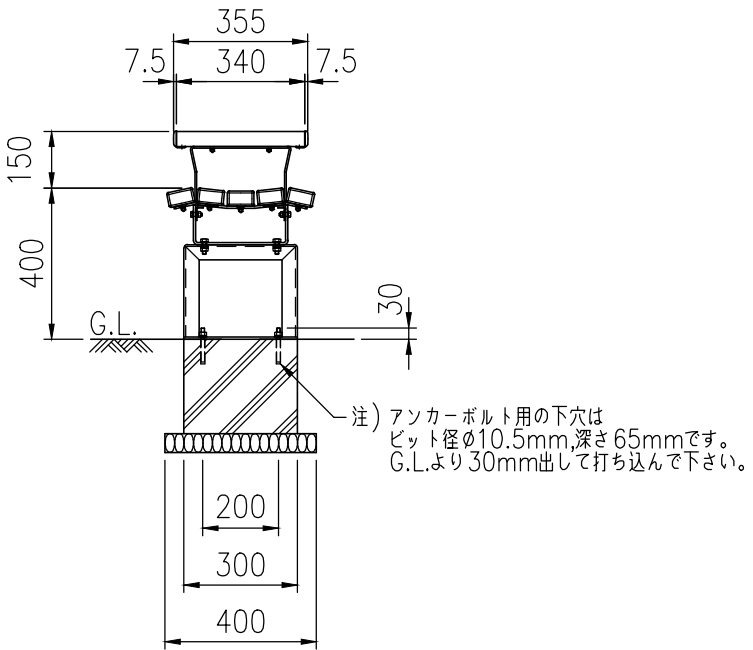
側面図(S=1/20)
