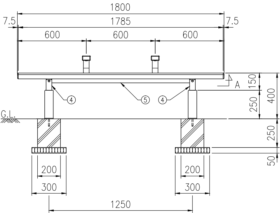
正面図(S=1/20)
