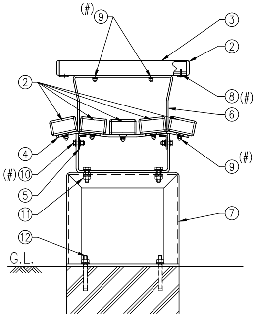
組付詳細図(S=1/10)
