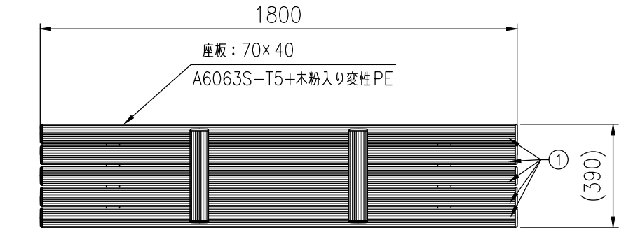
平面図(S=1/20)
