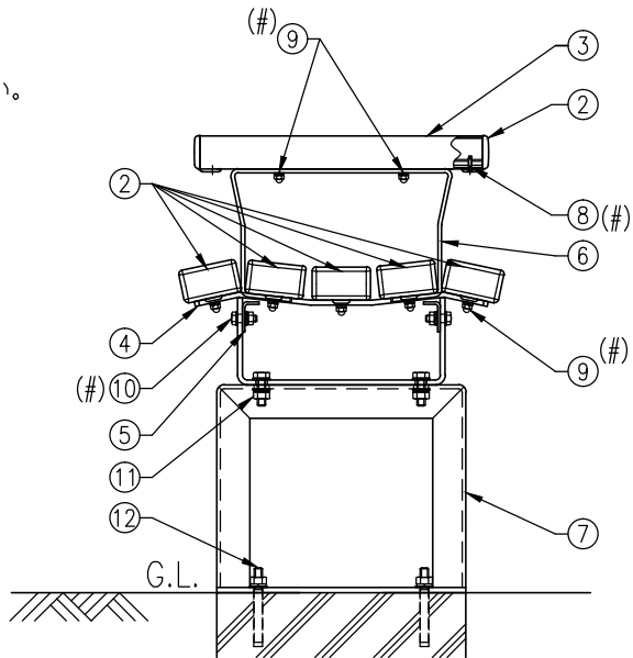
組付詳細図(S=1/10)
