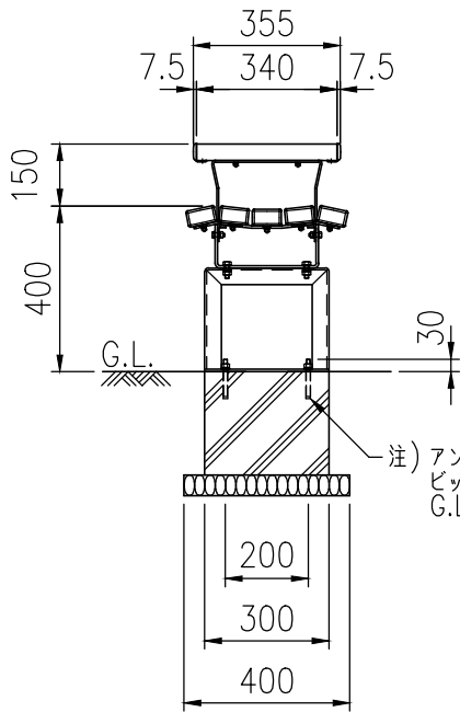
側面図(S=1/20)
