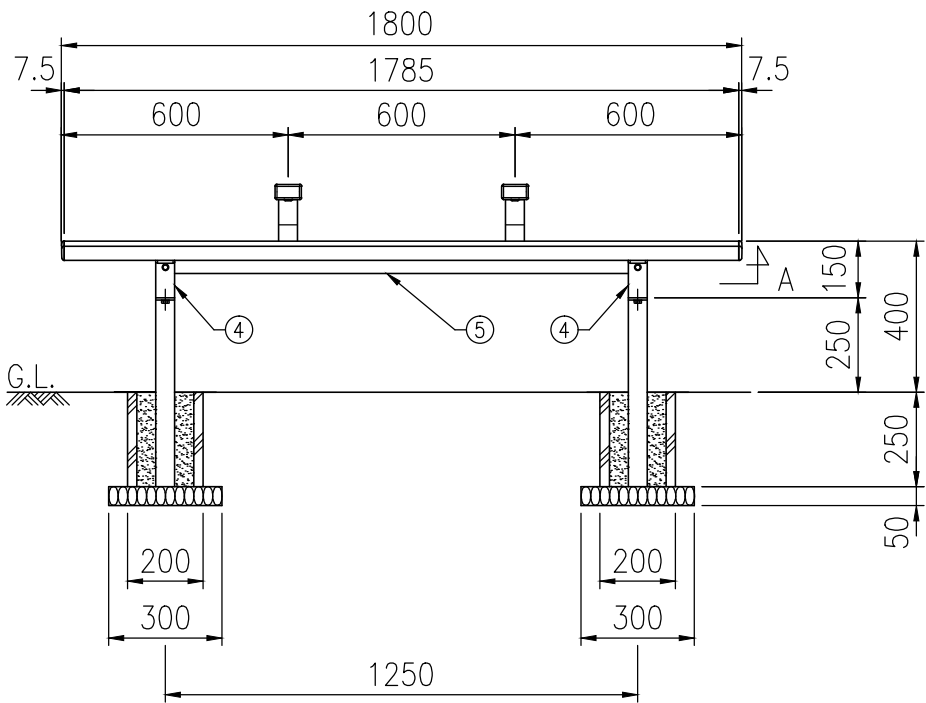
正面図(S=1/20)
