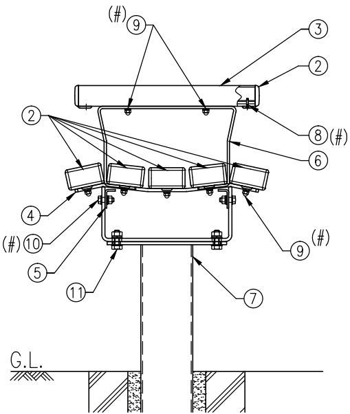
組付詳細図(S=1/10)
