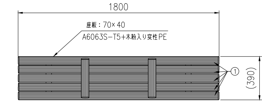
平面図(S=1/20)
