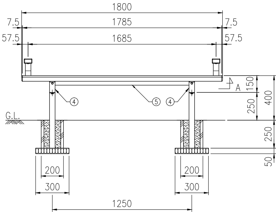
正面図(S=1/20)
