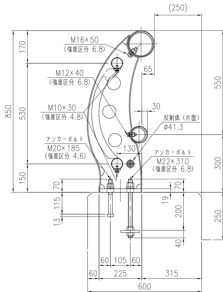
支柱図
