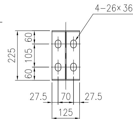
A 矢 視 図
