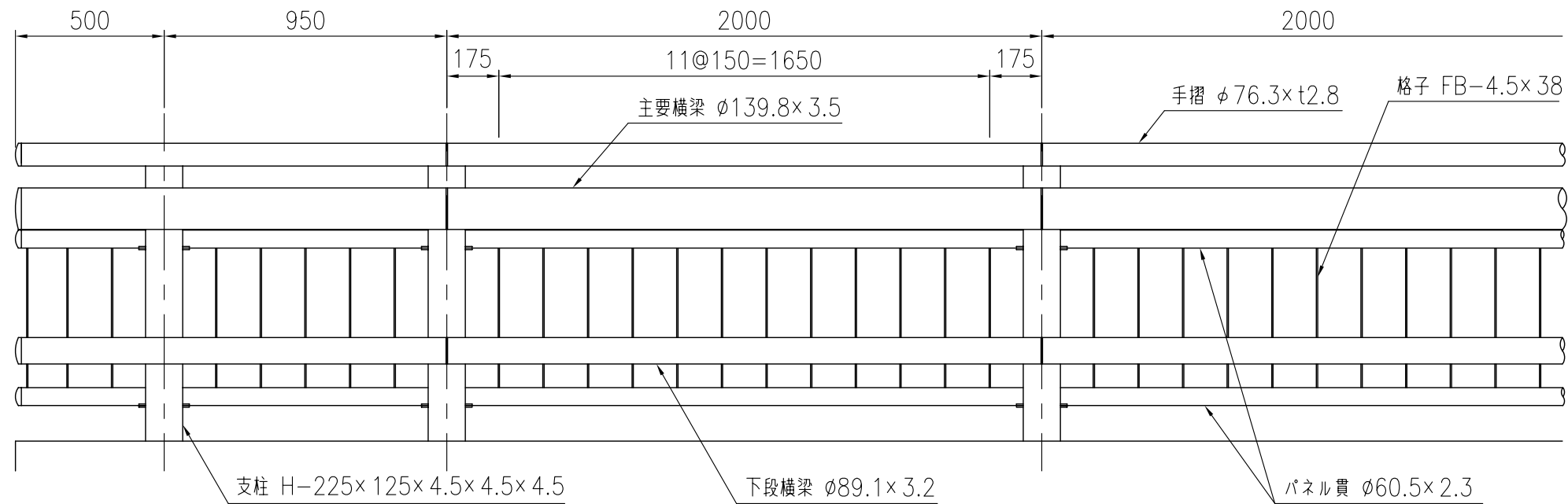
設置図
