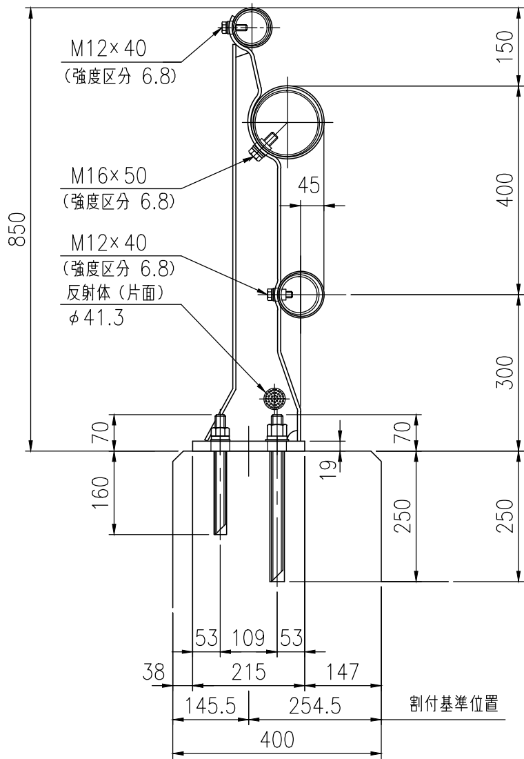
支柱図
