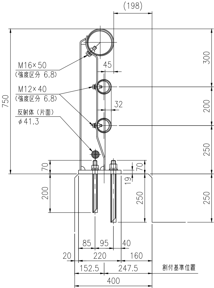
支柱図
