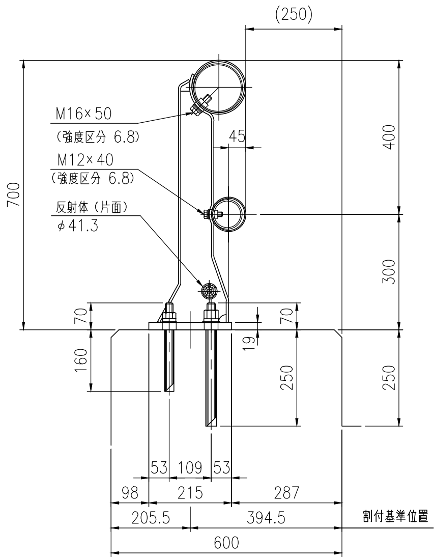
支柱図
