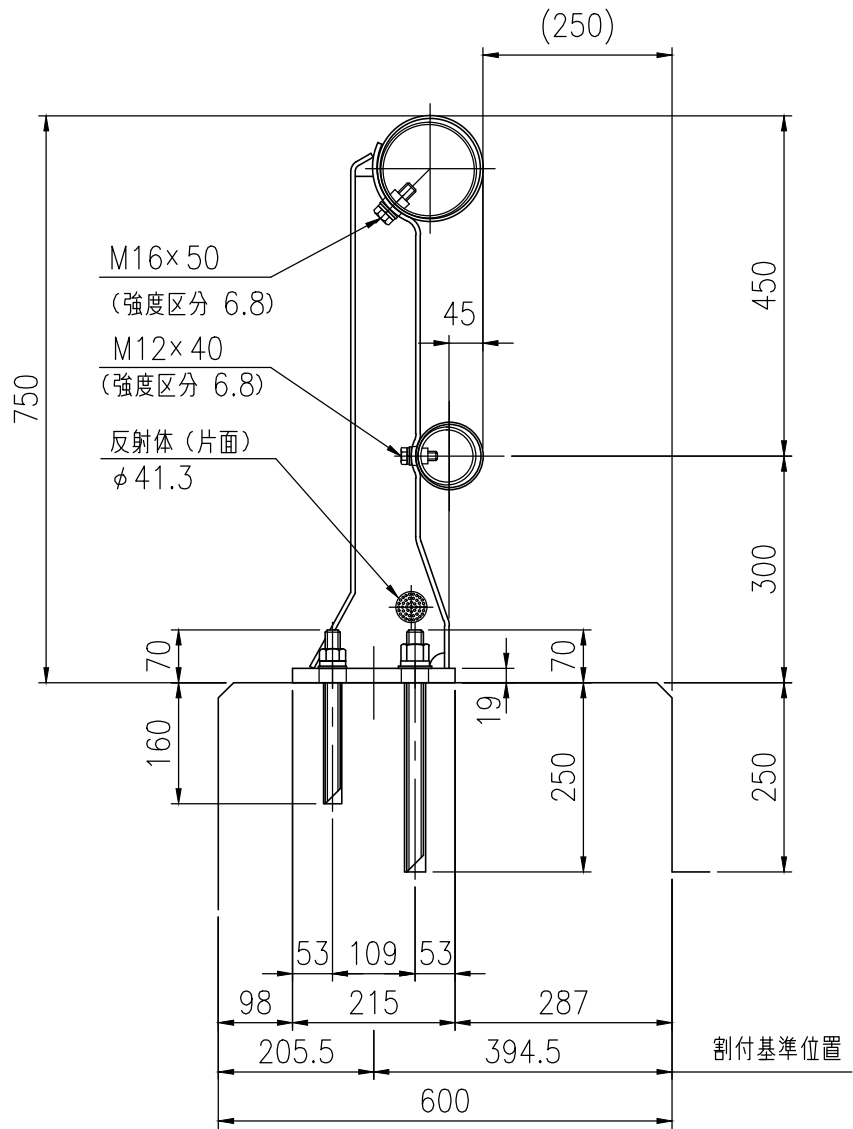
支柱図
