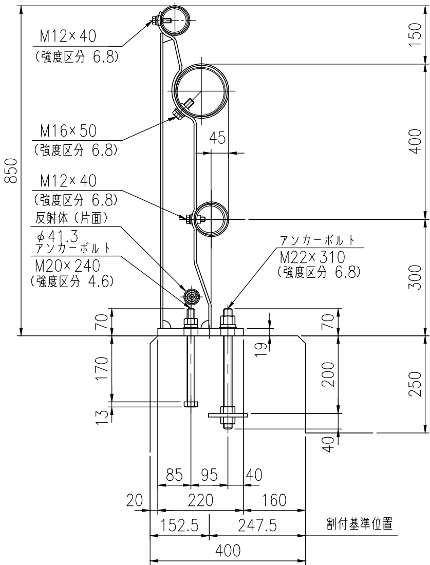
支柱図
