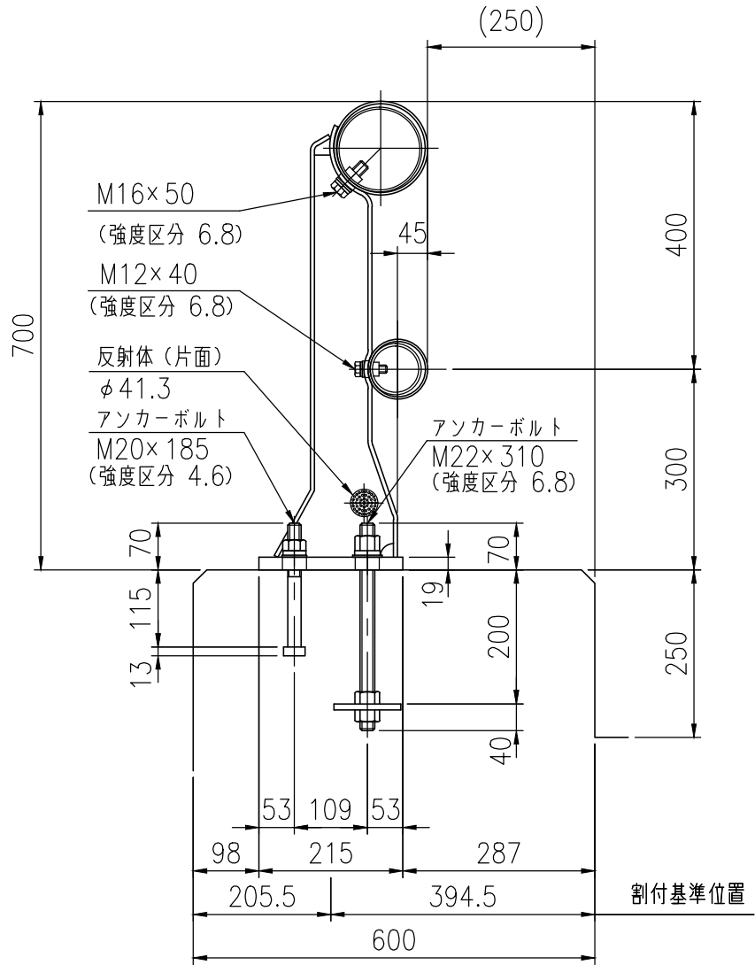
支柱図
