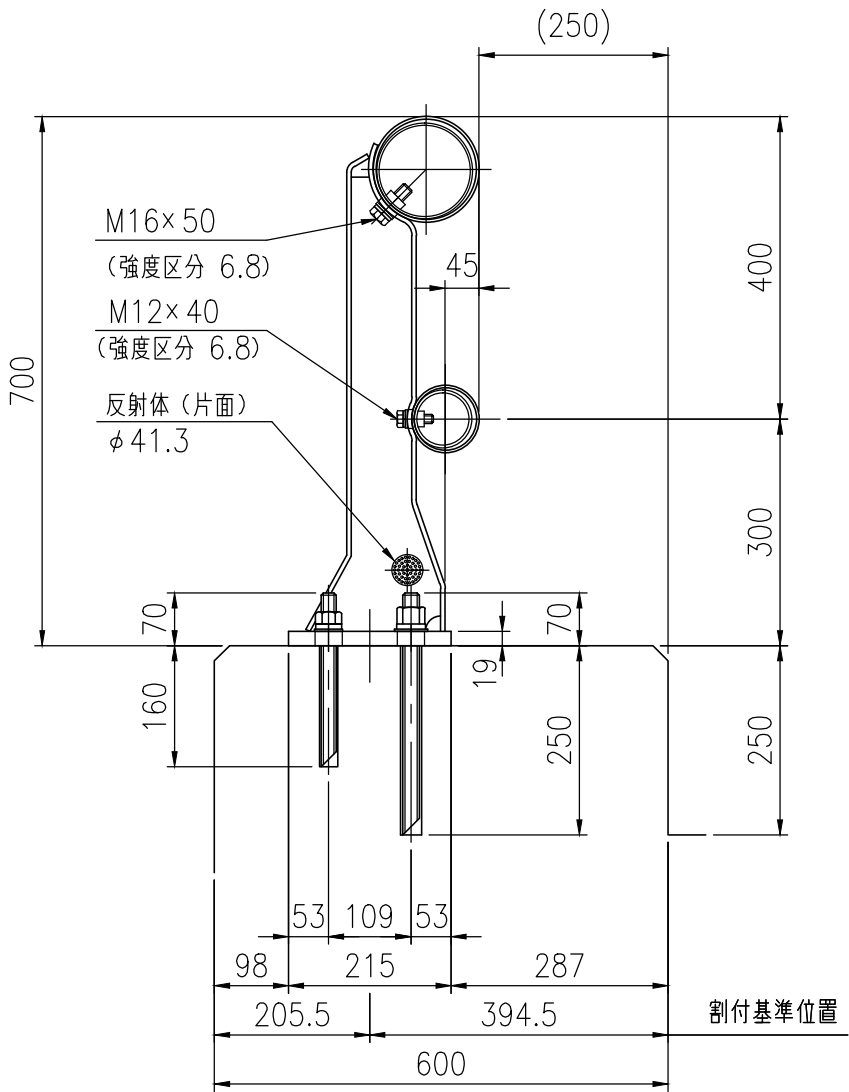
支柱図
