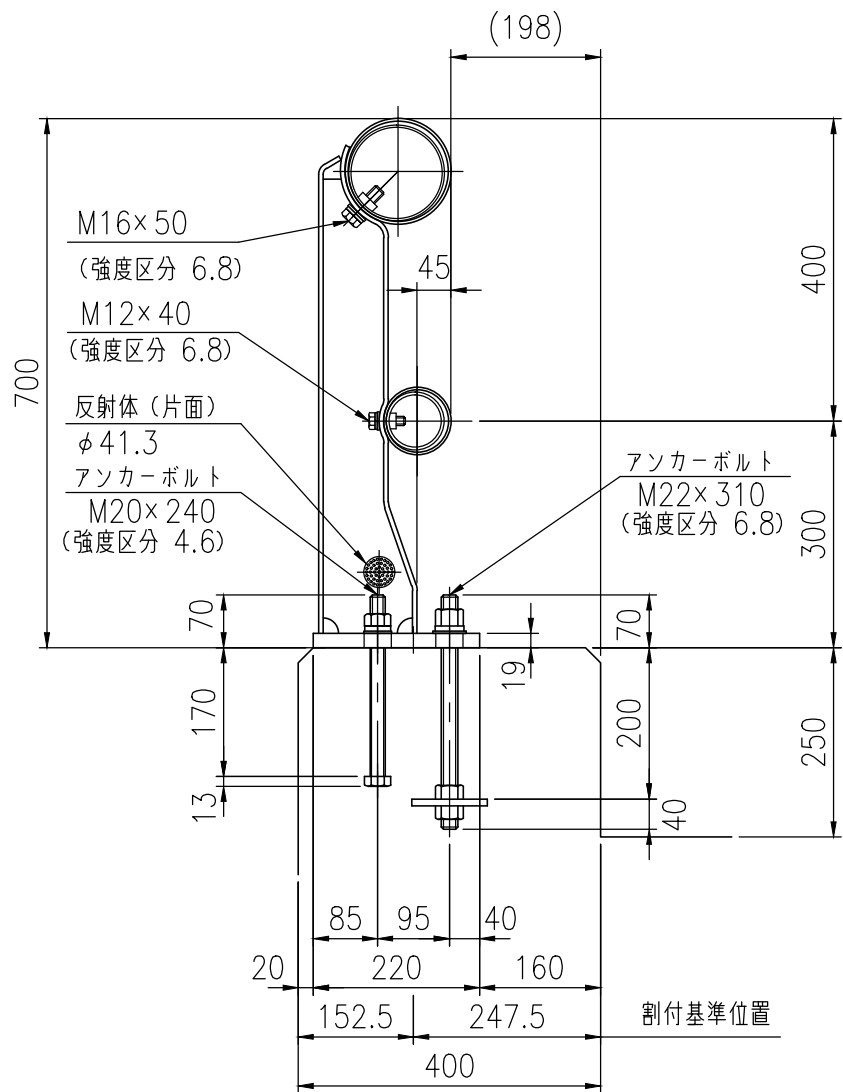
支柱図
