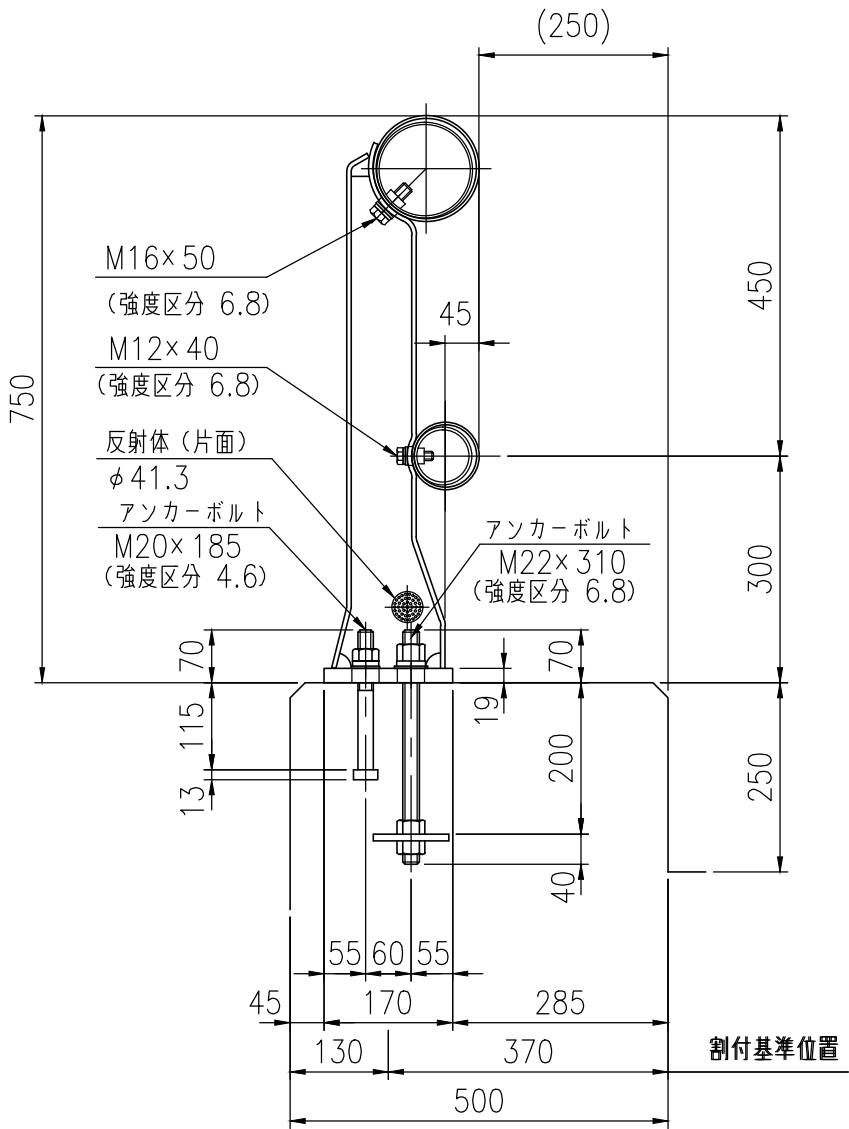
支柱図
