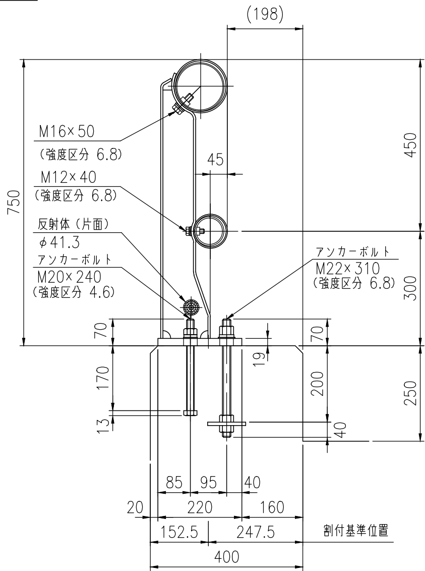
支柱図
