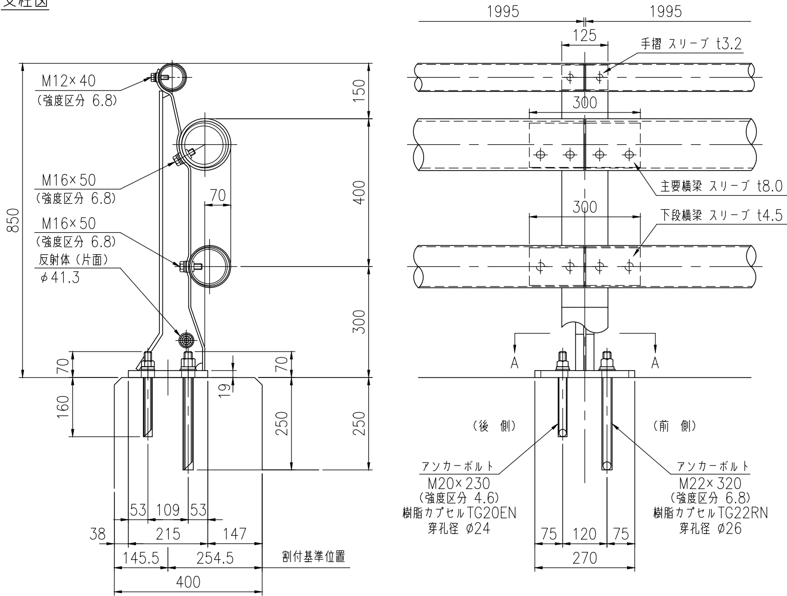
支柱図
