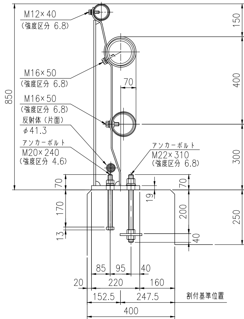
支柱図
